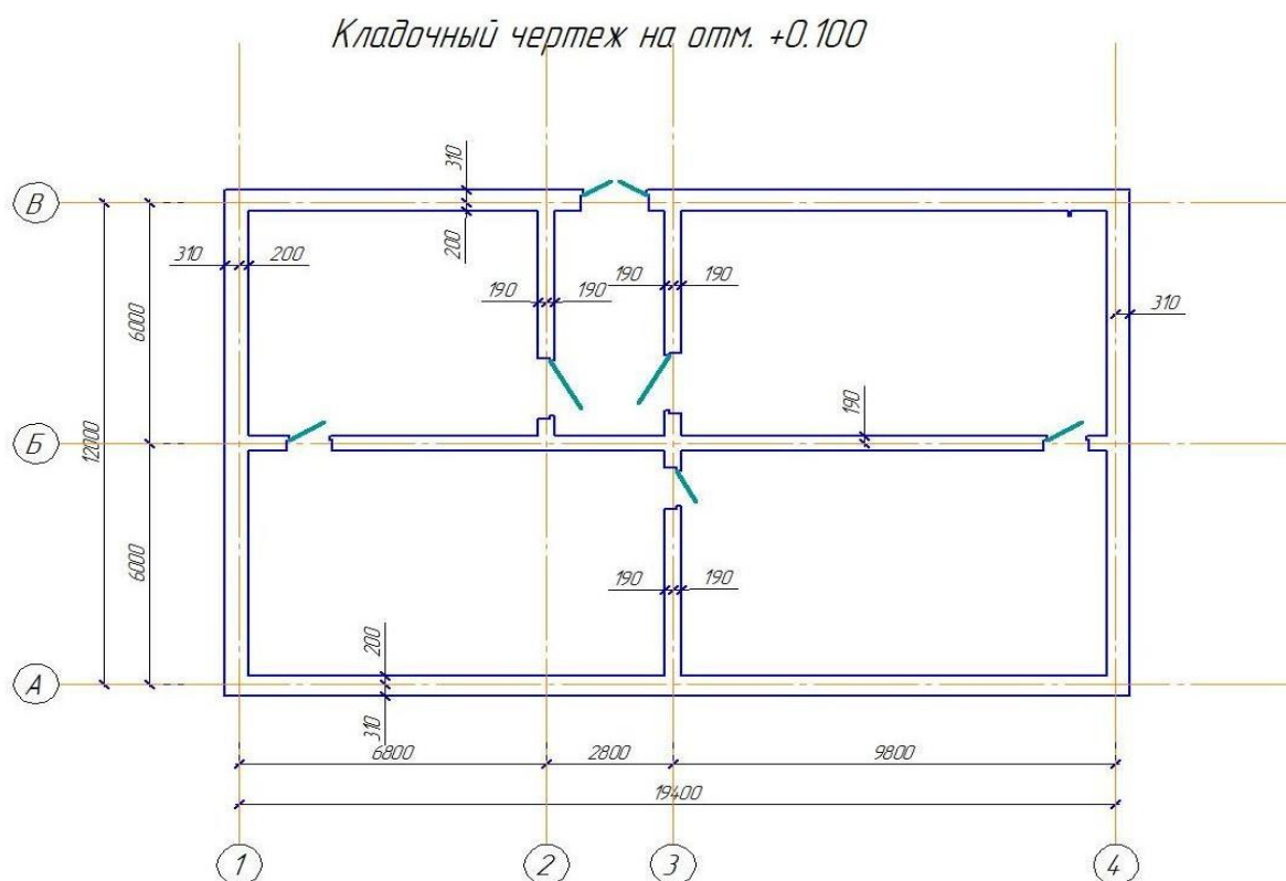
Рисунок 1. Кладочный чертеж
